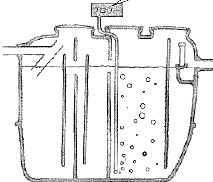
浄化槽
