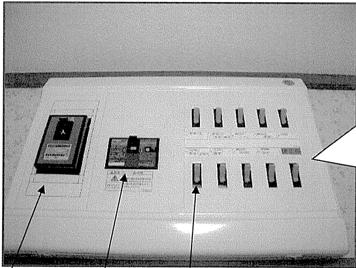
アンペアブレーカー 漏電遮断器 配線用遮断器
