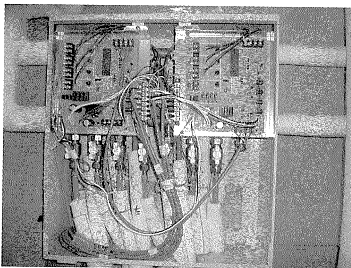
室外機 温水（不凍液）を温めます ヘッダー 温水を各部屋に分岐して送ります
