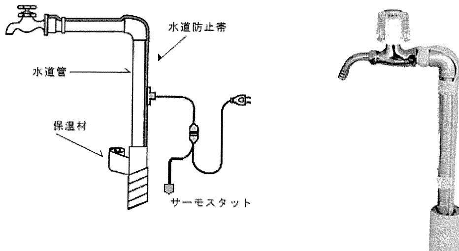
水道凍結防止帯（オートトレース）の実物写真
